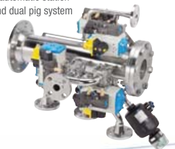
Empfangsstation Manuelle Betätigung, vollautomatisierte Stationen für Einmolch- und Zweimolchsysteme
