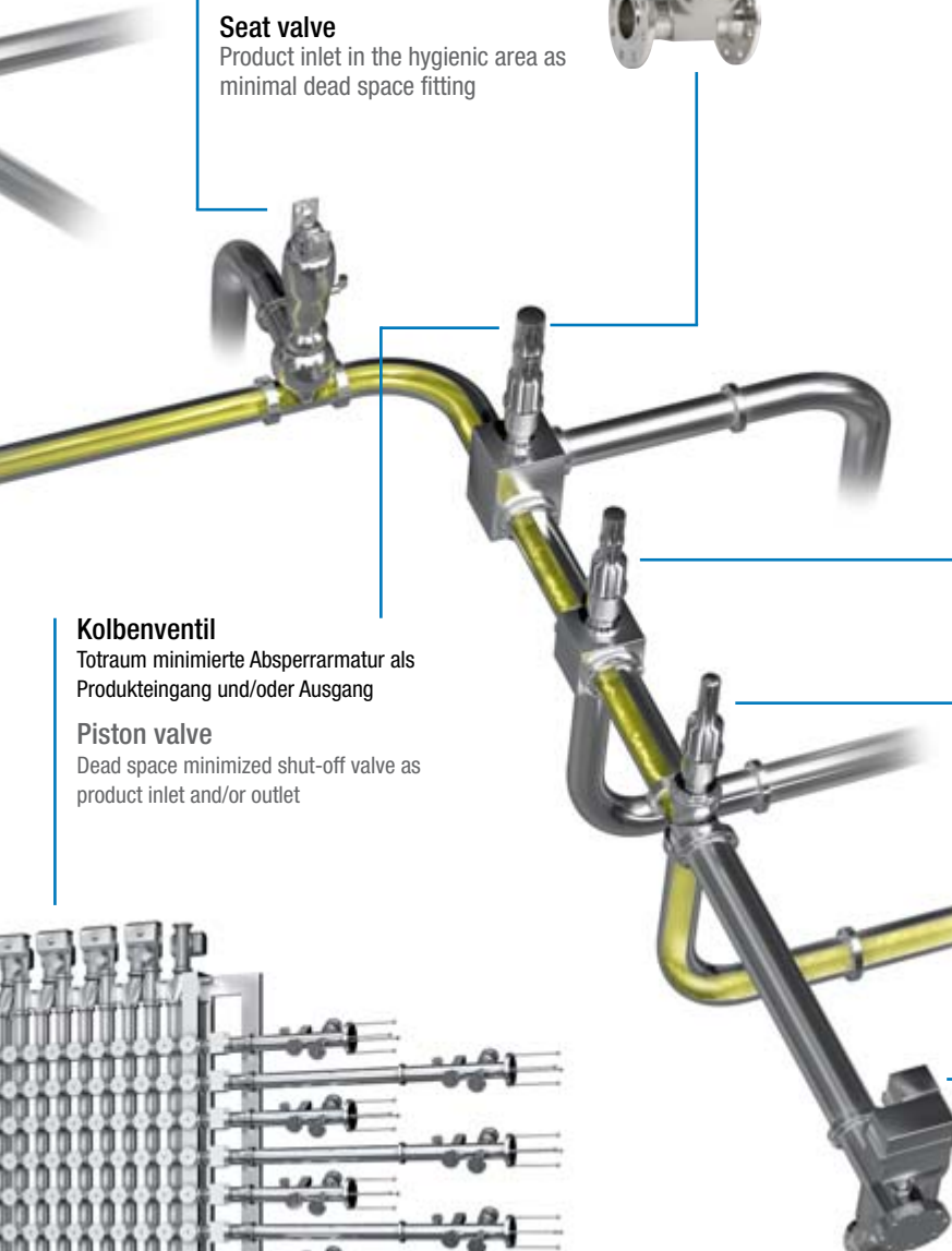
Sitzventil Produkteingang im Hygienebereich als tottraumarme Armatur
